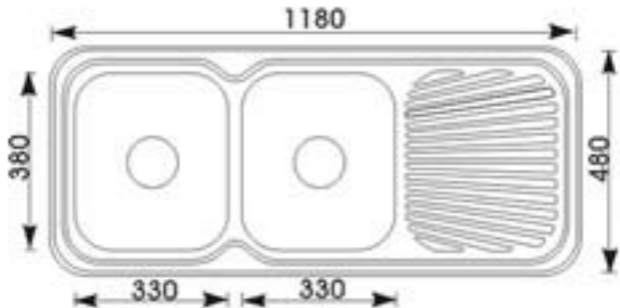
NH359CF(1180×480×170mm)
